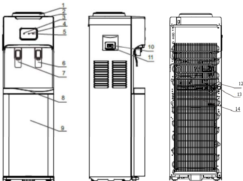
Рис. 1. Схема аппарата V115C
